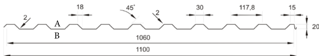
A-Pozitiv-tip ACOPERIS
